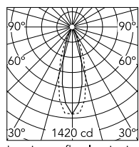
Luminous flux luminaire 523 lm
