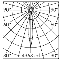
Luminous flux luminaire 387 lm
