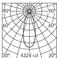
Luminous flux luminaire 2068 lm
