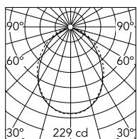
Luminous flux luminaire 491 lm
