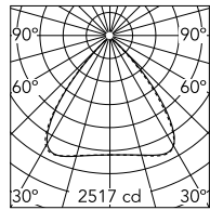
Luminous flux luminaire 3801 lm
